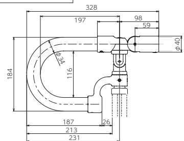
商品寸法図
