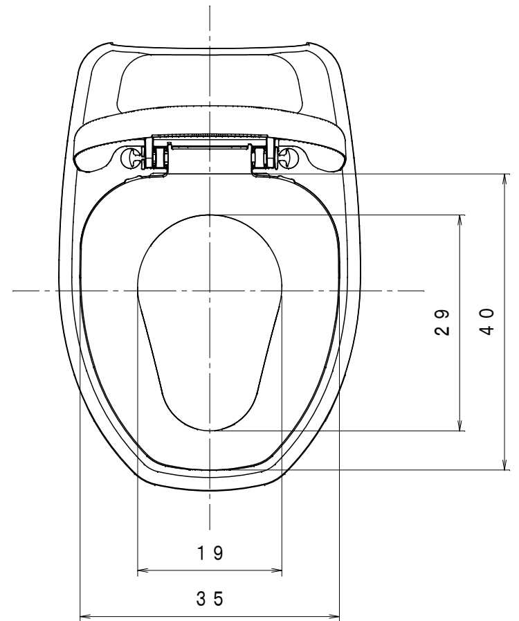
標準便座
