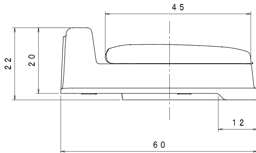
側面
