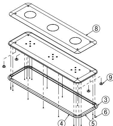
AT-CRベースプレートS
