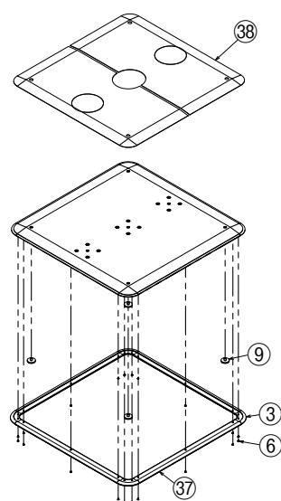
AT-CRベースプレートM
