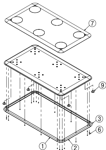
AT-CRベースプレートN
